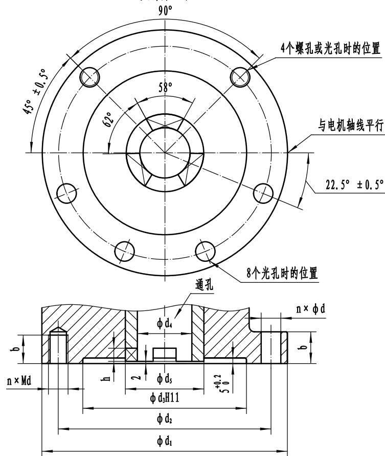
安装尺寸
