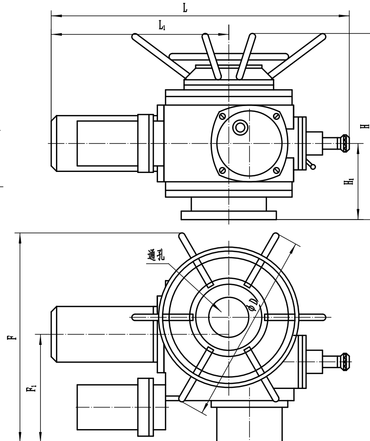
外形尺寸
