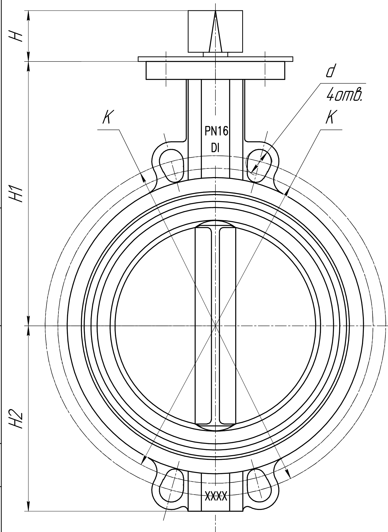
Основные габаритные и присоединительные размеры, мм
