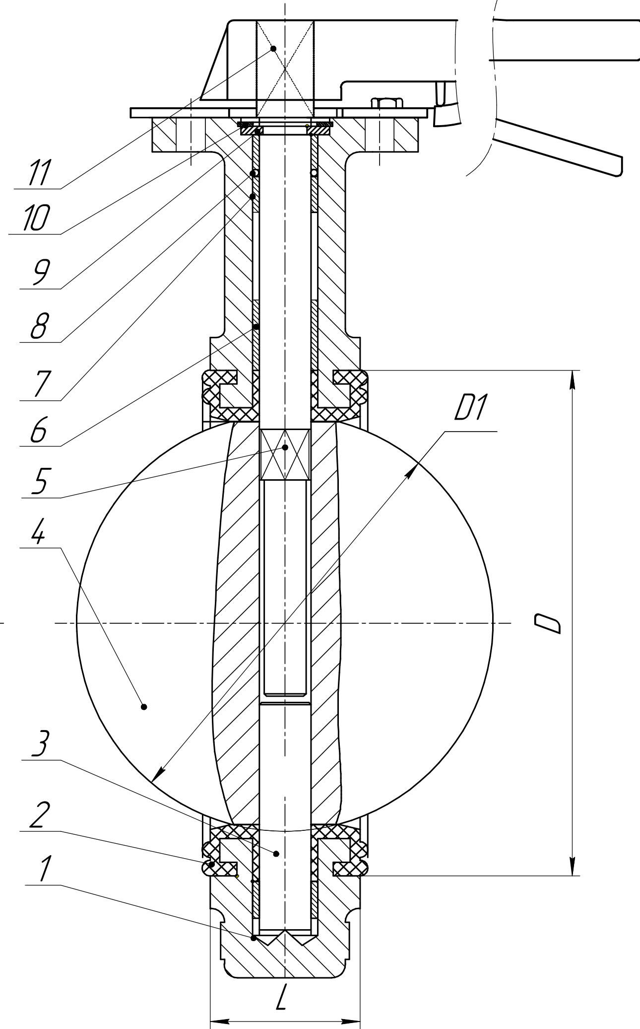
Основные габаритные и присоединительные размеры, мм
